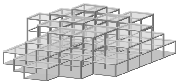
Fig. 2 Axonometrie der Struktur aus dem 3D-Modell. Overview of the structure from the 3D model.
