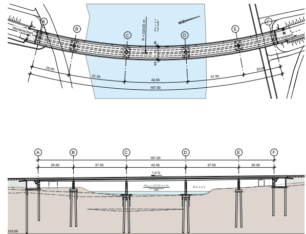
Fig. 3 Reussbrücke, Längsschnitt. Reuss bridge, longitudinal section.
