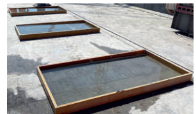
Fig. 9 Dichtigkeitsprüfung der Stossfuge. Tightness test of the butt joint.
