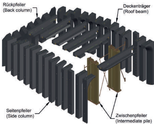
Fig. 6 3D-Darstellung der vorfabrizierten Elemente der Haube. 3D-view of the cap precast elements.
