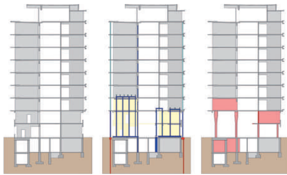
Fig. 10 Umbaukonzept Foyer: Bestand/Notspriessung und Abbruch/Neubau.
