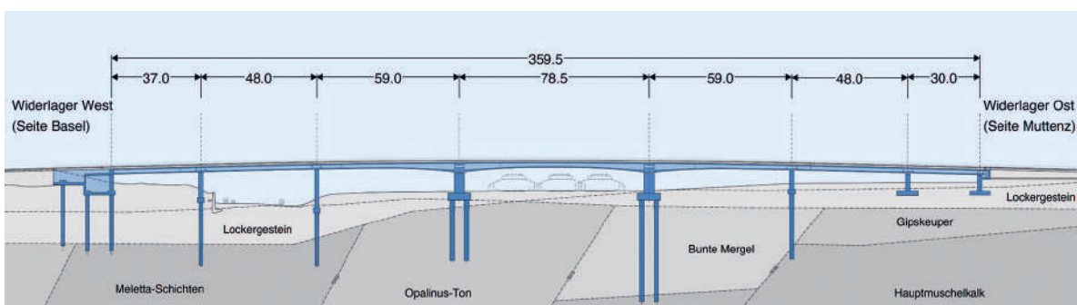
Fig. 3 Längsschnitt. Longitudinal section.
