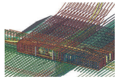
Fig. 10 Detail der Bewehrung der Wendeltreppe. Detail of the reinforcement of the helical stair.
