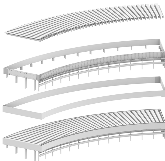
Fig. 5 Tragsystem für das Dach des Erweiterungsbaus der Unithèque. Structural system for the roof of the Unithèque extension.
