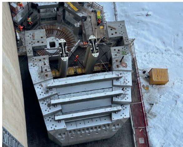
Fig. 7 Ansicht der vorfabrizierten Elemente der Haube. View of the cap precast elements.
